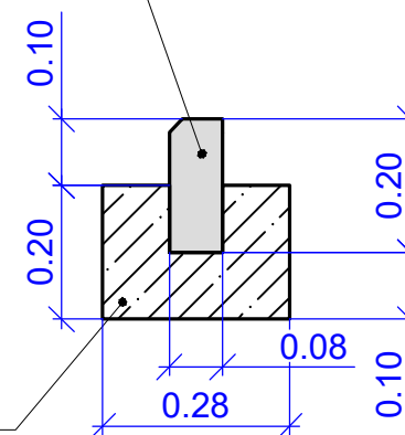
Схема монтажа бордюрного камня
